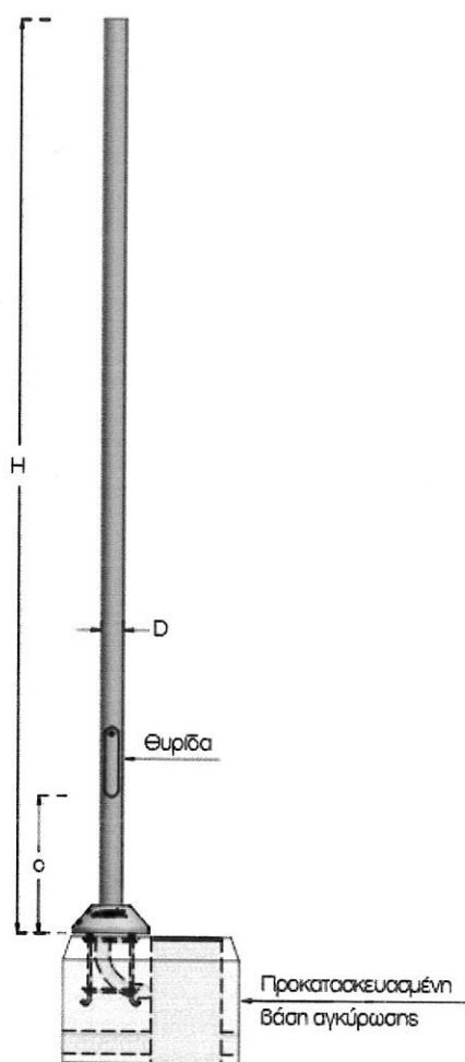
Εικόνα 3. Ενδεικτικό σχέδιο ιστού (περιλαμβάνεται κατάλληλη διάταξη κολουροκωνικής μορφής που καλύπτει τις ντίζες και τα περικόχλια της βάσης)
