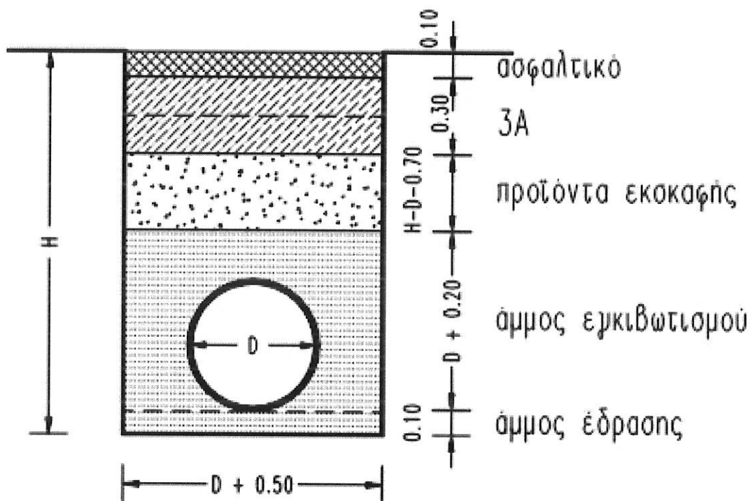
Εικόνα 2. Ενδεικτική τομή σκάμματος διέλευσης καλωδίων.
